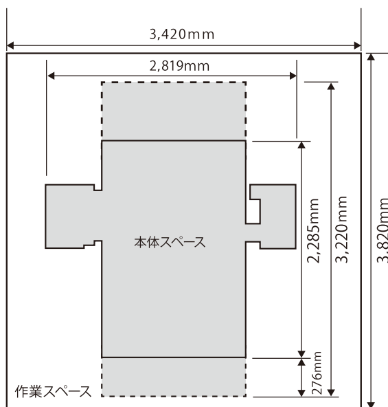
外観寸法イメージ
